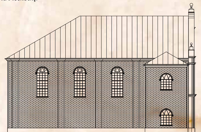
Synagoga w Dynowie - rekonstrukcja. Elewacja północna. Wykonała Lidia Tobiasz na podstawie szkiców opracowanych przez Michała Piechotkę.
