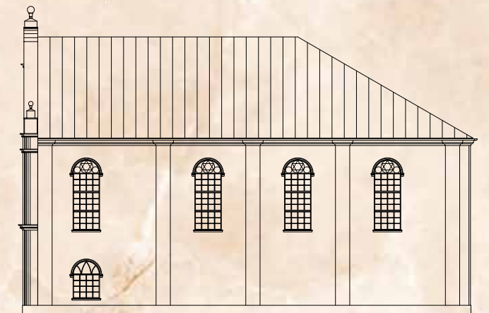
Synagoga w Dynowie - rekonstrukcja. Elewacja południowa. Wykonała Lidia Tobiasz na podstawie szkiców opracowanych przez Michała Piechotkę.
