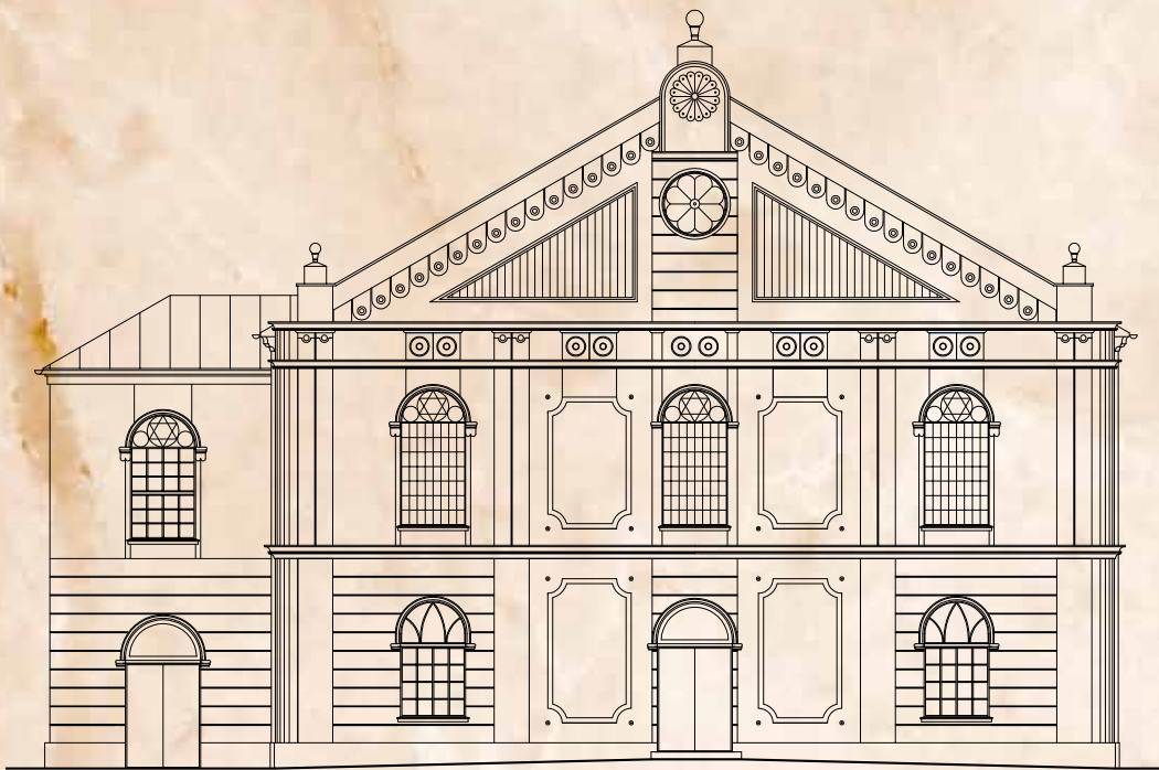
Synagoga w Dynowie – rekonstrukcja. Elewacja zachodnia - frontowa. Wykonała Lidia Tobiasz na podstawie szkiców opracowanych przez Michała Piechotkę.
