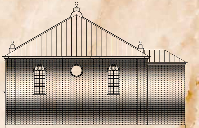
Synagoga w Dynowie - rekonstrukcja. Elewacja wschodnia. Wykonała Lidia Tobiasz na podstawie szkiców opracowanych przez Michała Piechotkę.
